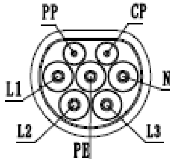
Ladestation Stecker – Typ 2
