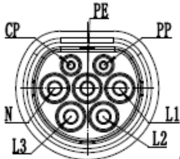
E-Auto Stecker – Typ 2
